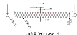
PCB布局 (PCB Layout)
